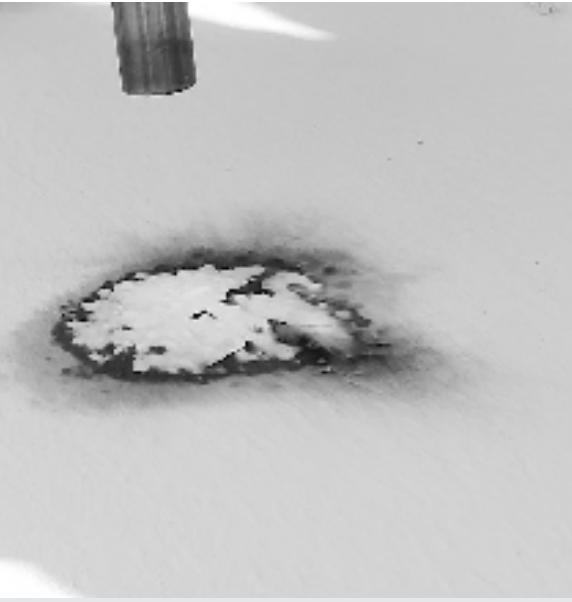
喷枪燃烧测试
