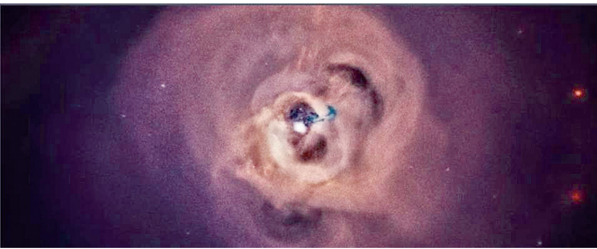
英仙座星系团,由钱德拉X射线天文台拍摄。
